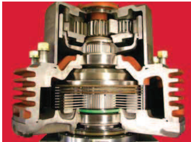
Sistema de freno de disco en aceite completamente cerrado
